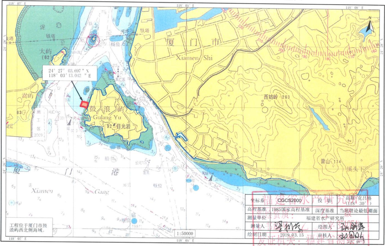
厦门鼓浪屿内厝澳码头扩建工程宗海位置图
