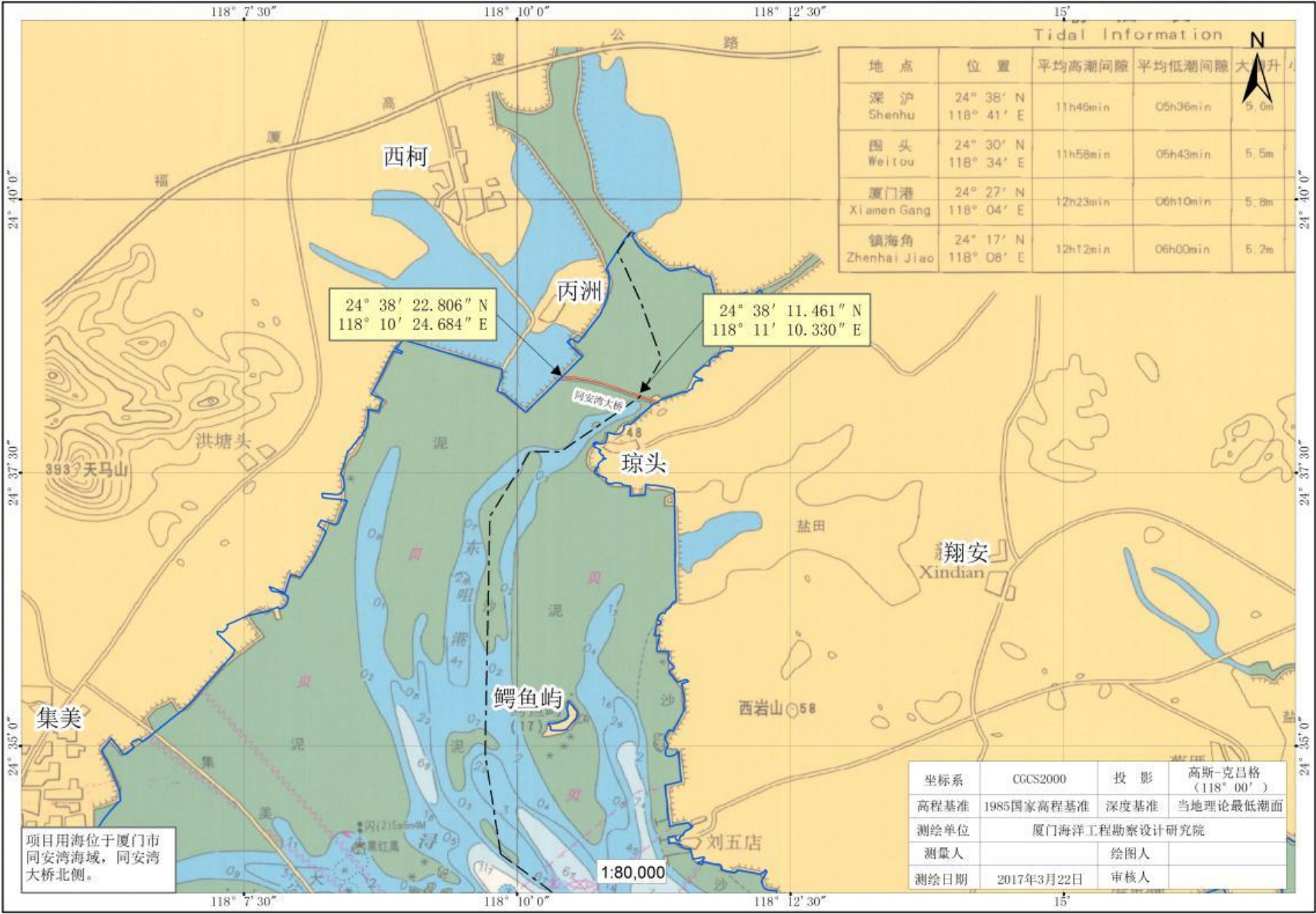
厦门市轨道交通4号线同安湾过海段工程宗海位置图
