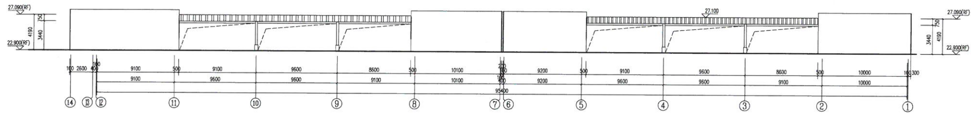
屋面分布式光伏北立面图 1:150
