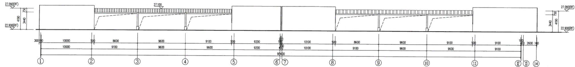
屋面分布式光伏南立面图 1:150
