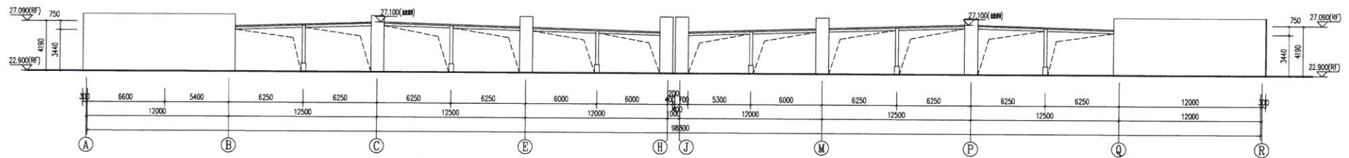
屋面分布式光伏东立面图 1:150
