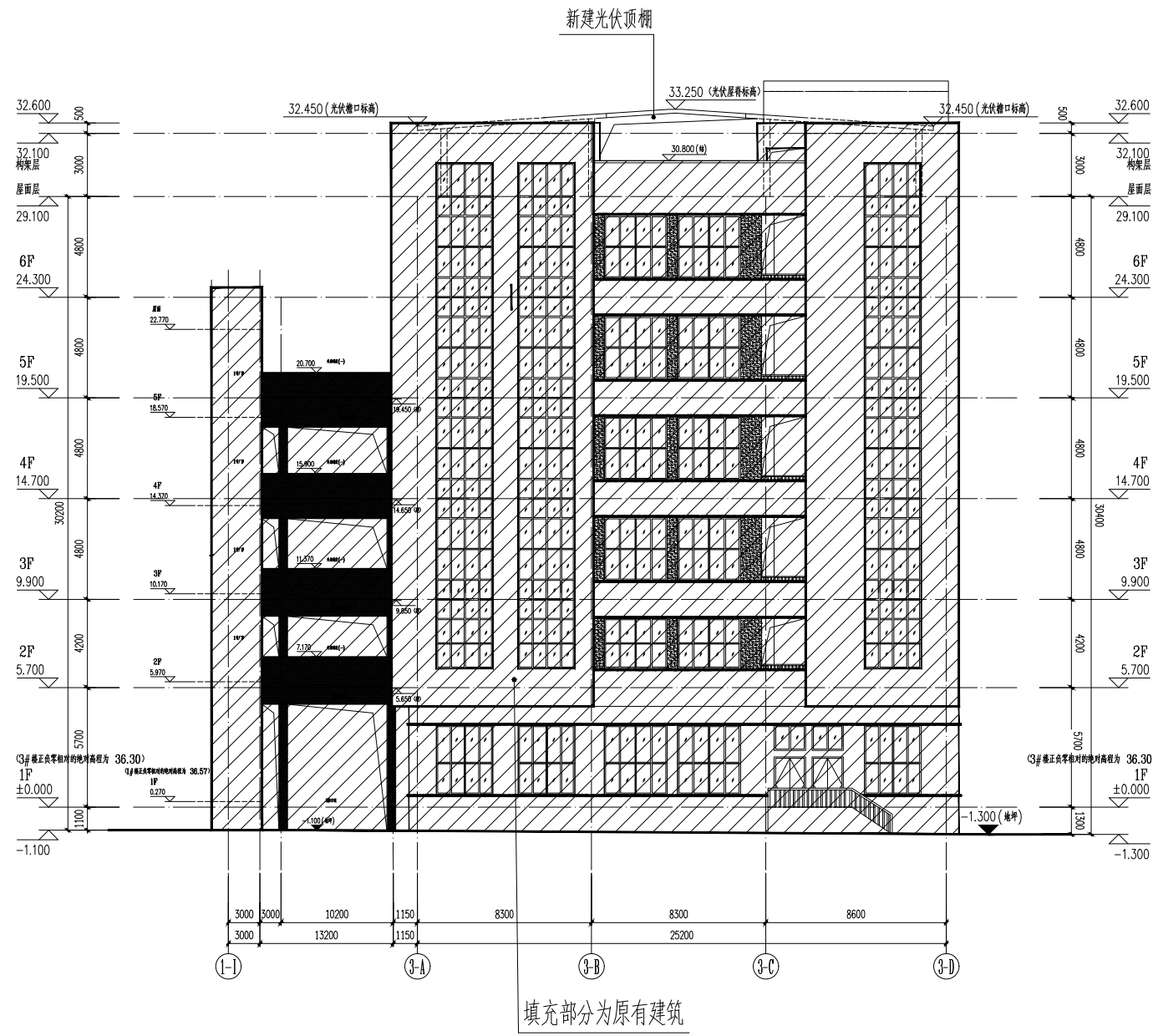
④~⑤轴立面图 1:100
