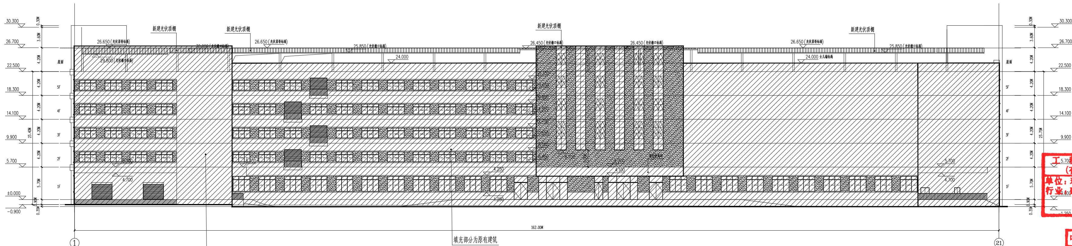
①-②轴立面图 1:200
