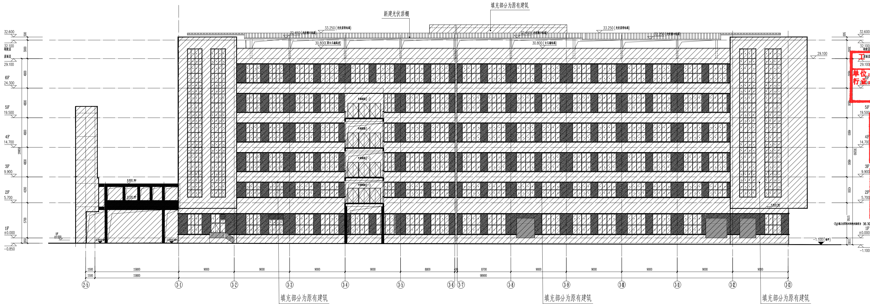
③~⑭轴立面图 1:100
