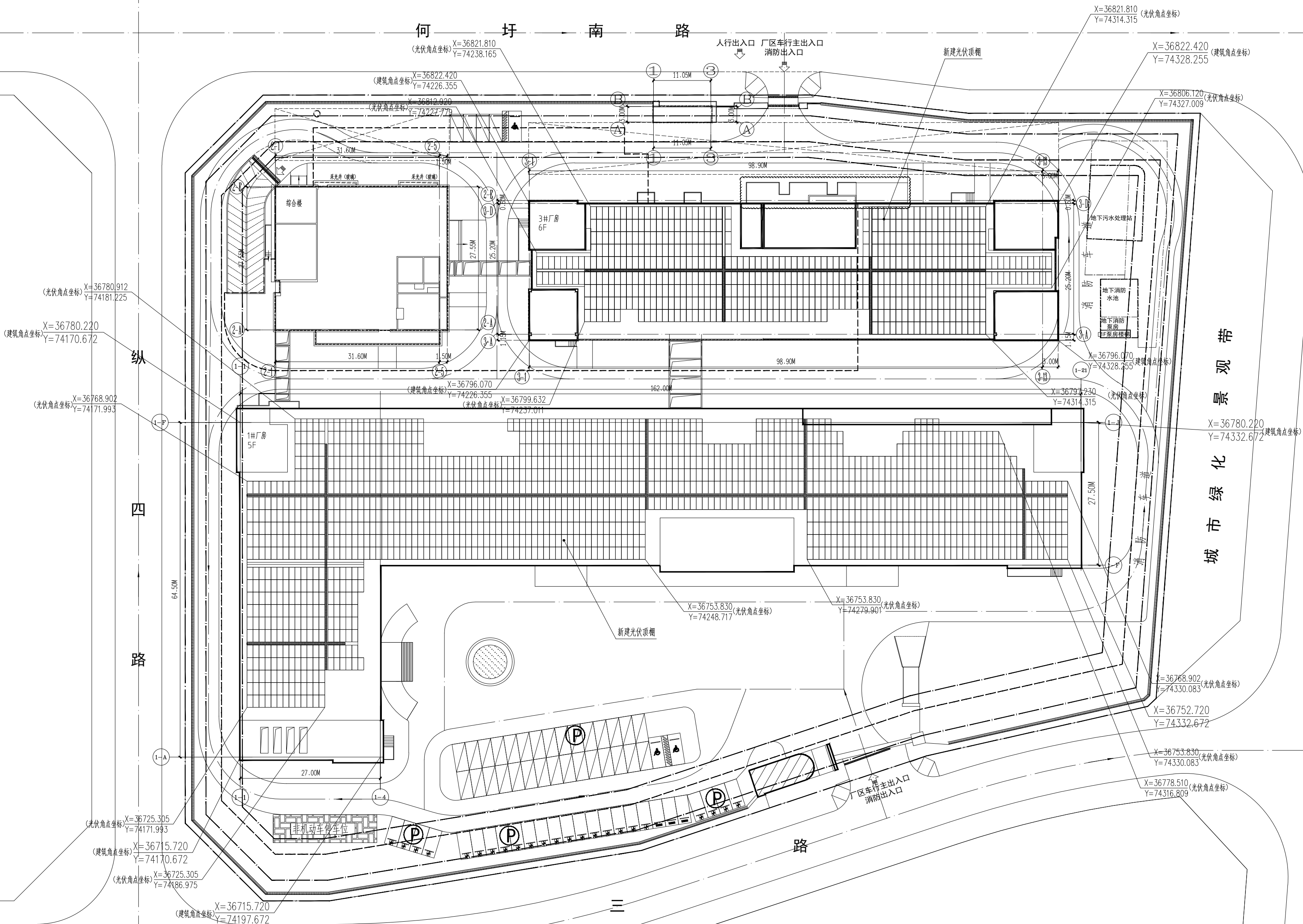
屋顶分布式光伏总平面布置示意图 1:400
