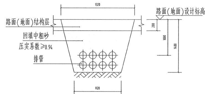
G6、G8 工井排管纵向断面图
