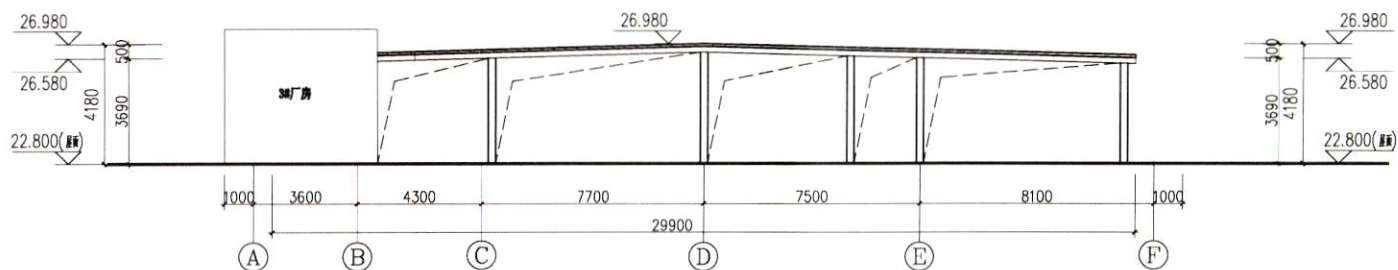
A~F轴立面图 1:125
