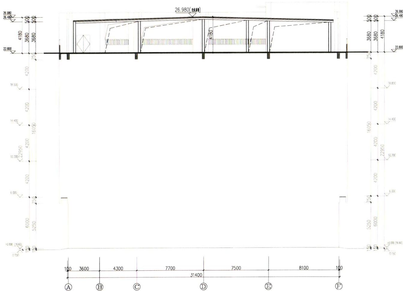
1-1剖面图 1:100
