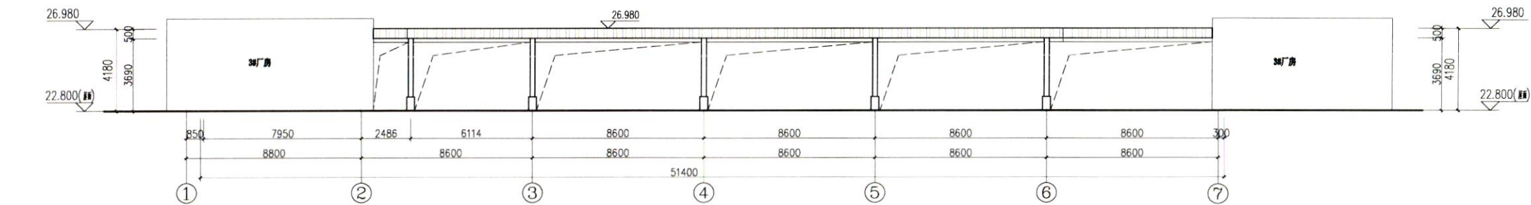
3#厂房 屋面分布式光伏南立面图 1:125
