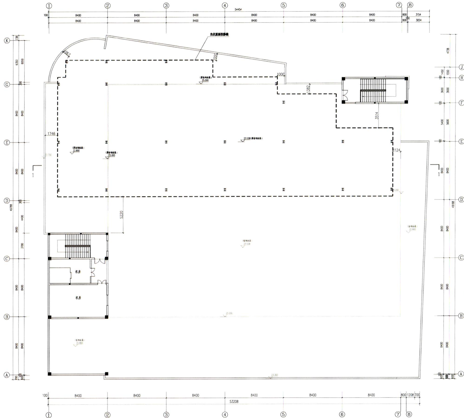
1#厂房屋顶分布式光伏底层平面图 1:125
