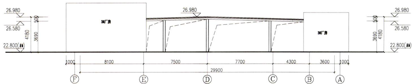
F~A轴立面图 1:125
