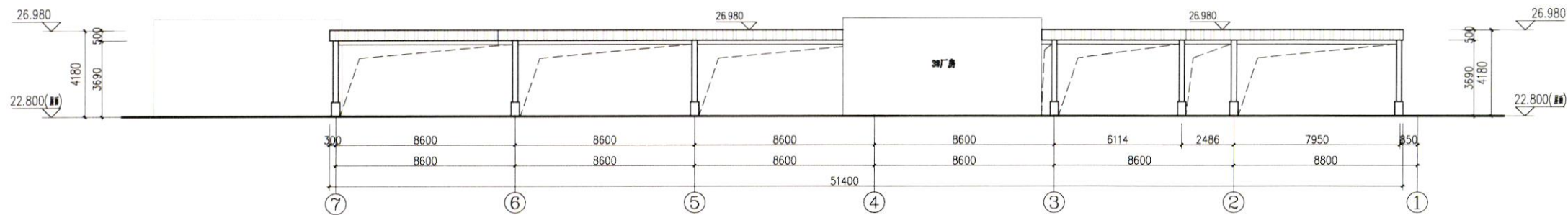
3#厂房 屋面分布式光伏北立面图 1:125
