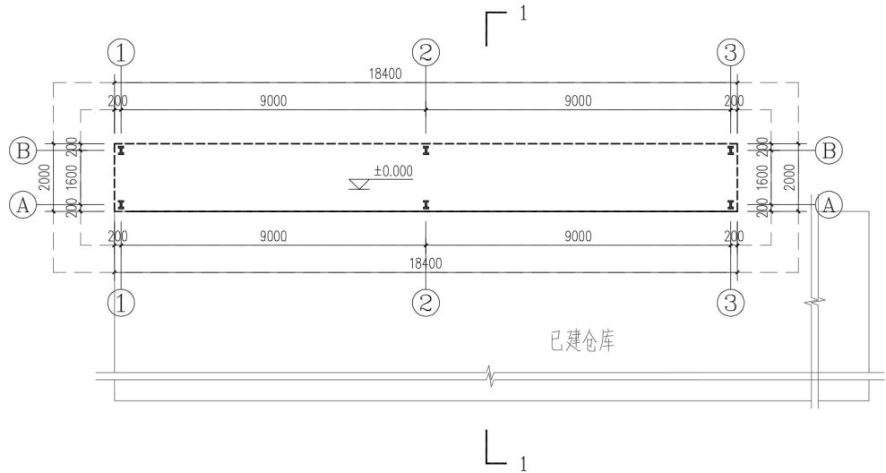
3#遮雨棚平面图 1:200
