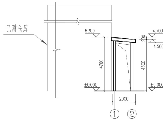
1-1剖面图 1:200
