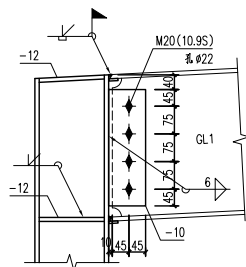
① GL 1 与刚架柱连接节点
