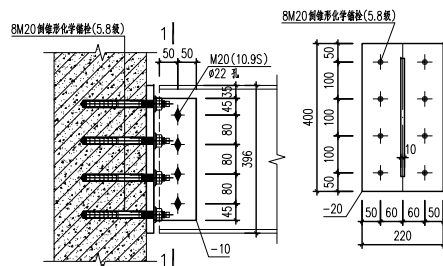
② GL1 与砼结构铰接节点
