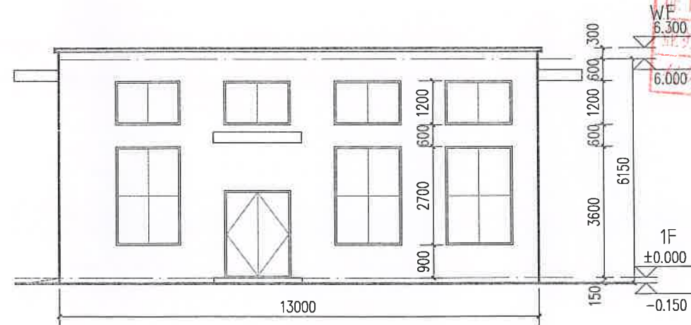
配电室南立面图 1:100
