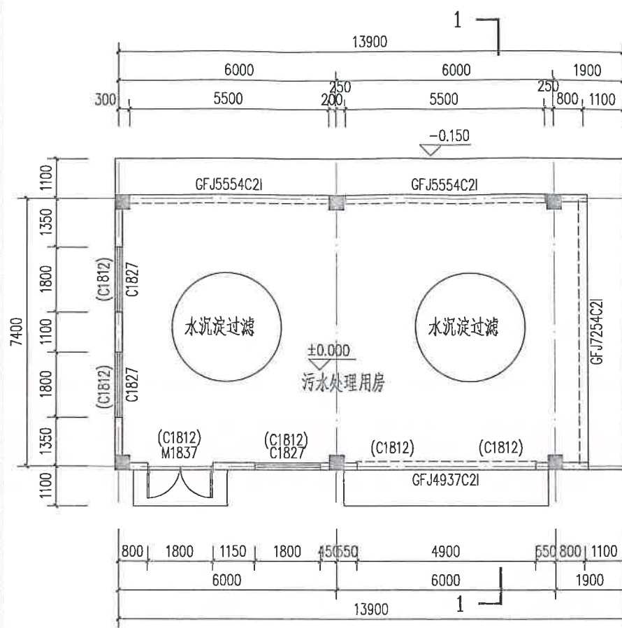
污水处理用房 一层平面图 1:100 污水处理用房面积99平方米
