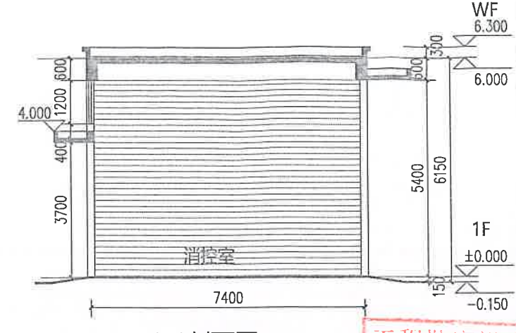
1-1剖面图 1:100
