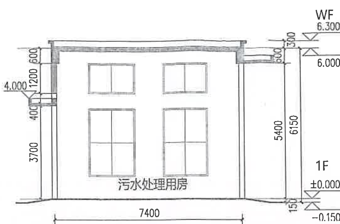
1-1剖面图 1:100
