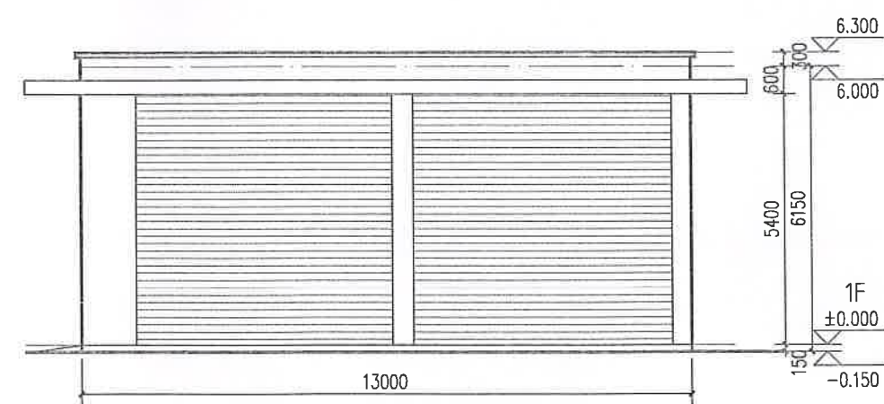
污水处理用房北立面图 1:100
