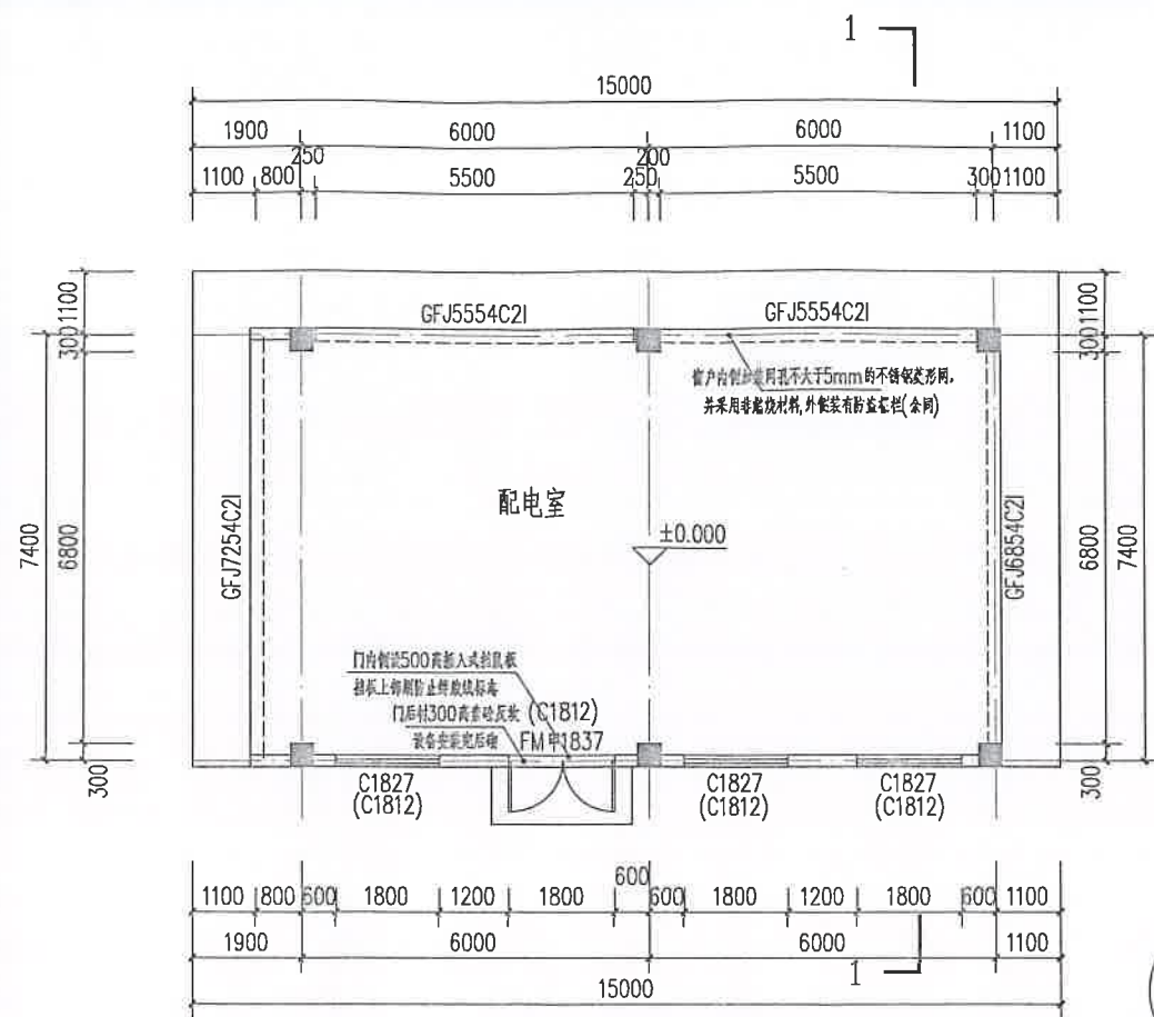
配电室 一层平面图:100
