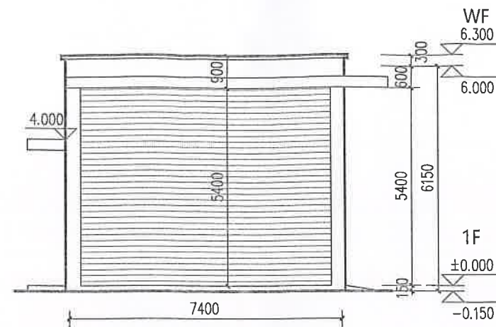
配电室东立面图 1:100
