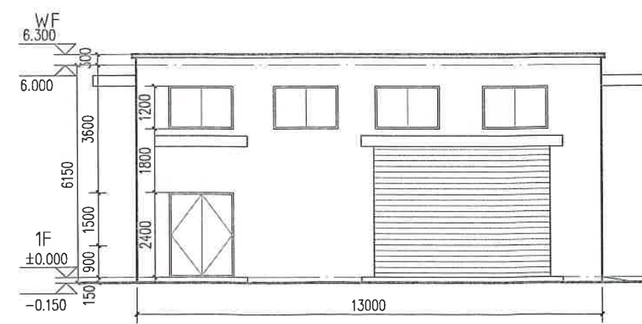
污水处理用房南立面图:100
