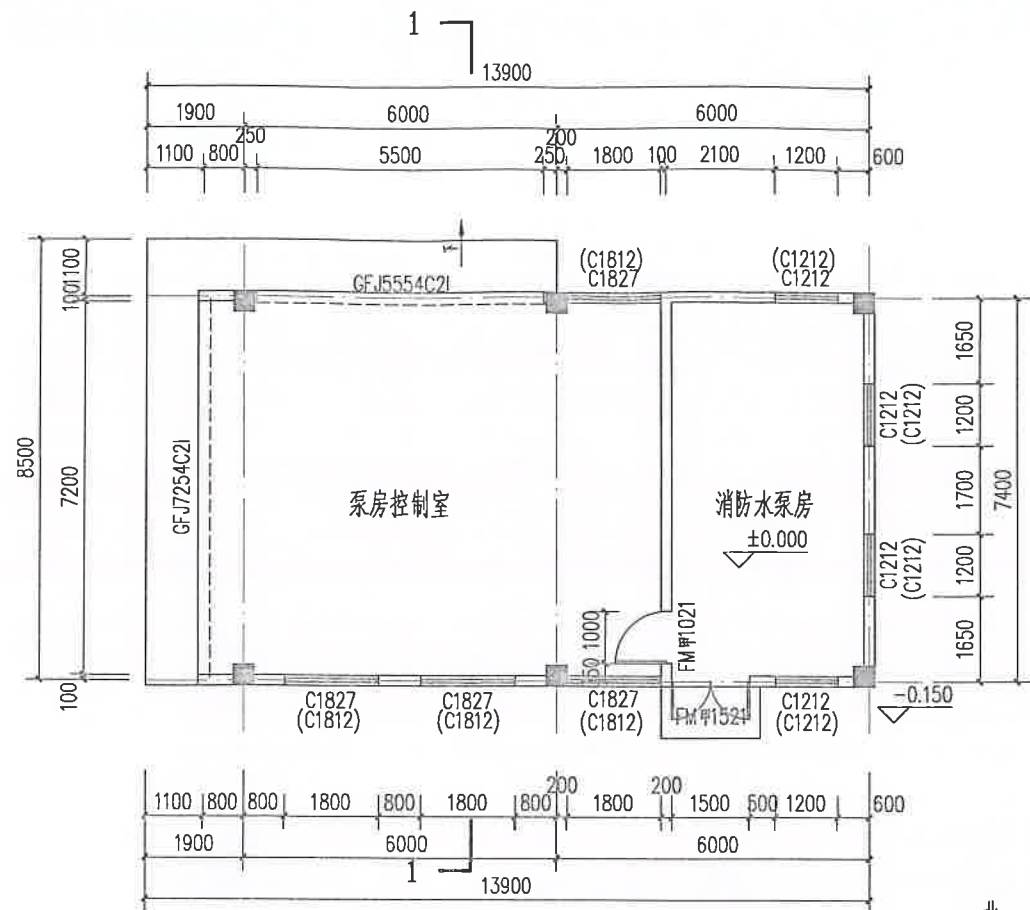
消防水泵房 一层平面图 1:100
