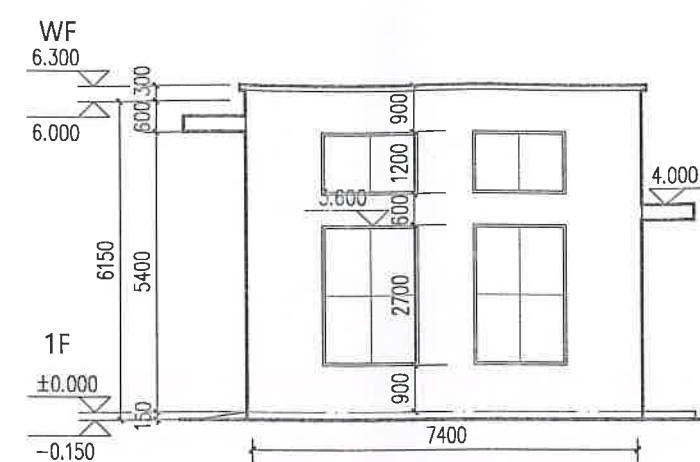
污水处理用房西立面图 1:100
