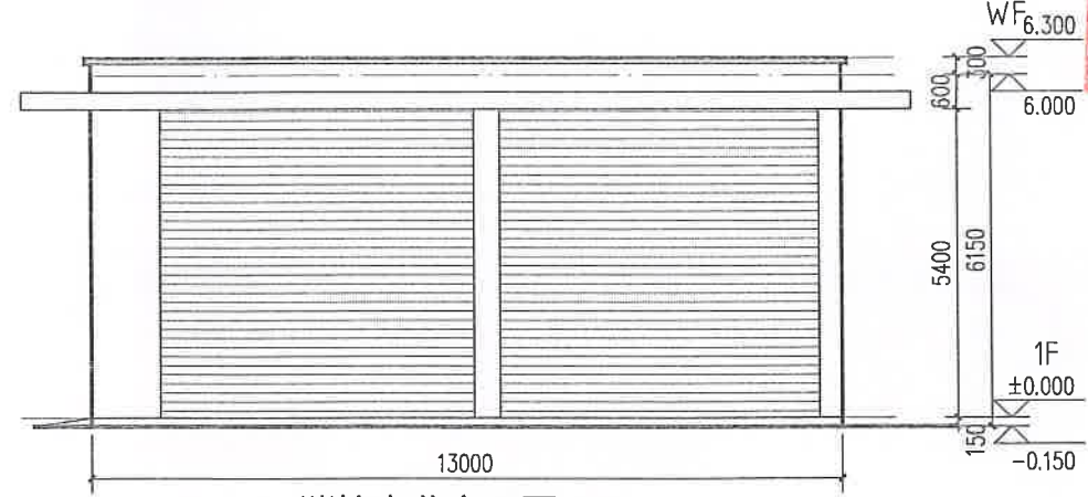
消控室北立面图 1:100
