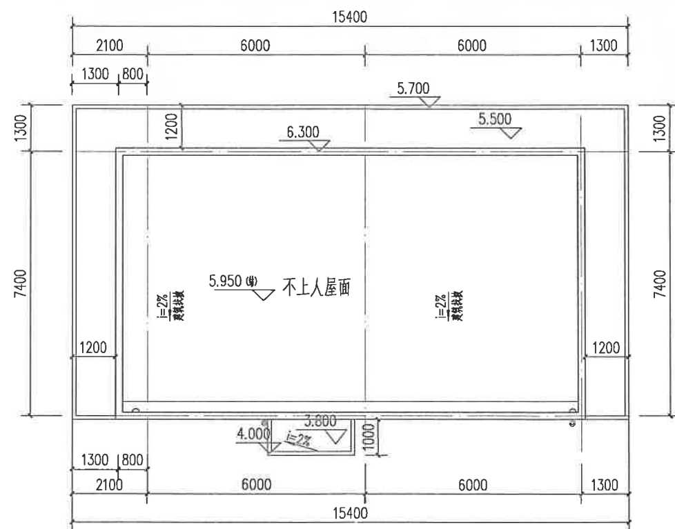
配电室 屋面层平面图 1:100
