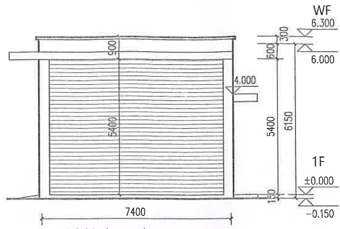
消控室 西立面图 1:100
