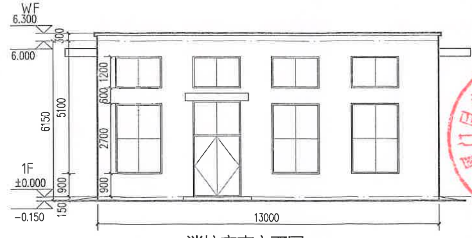
消控室南立面图 1:100
