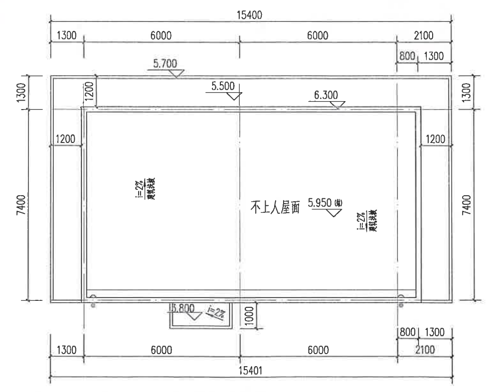
消控室 屋面层平面图 1:100
