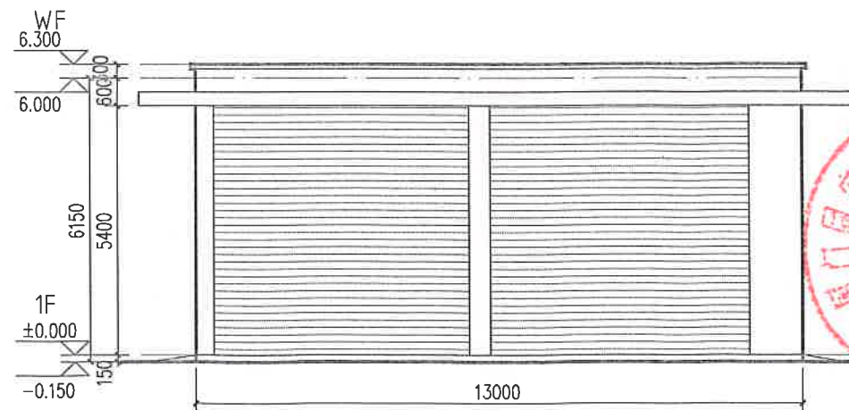
配电室北立面图 1:100
