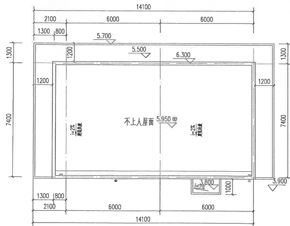
消防水泵房 屋面层平面图 1:100
