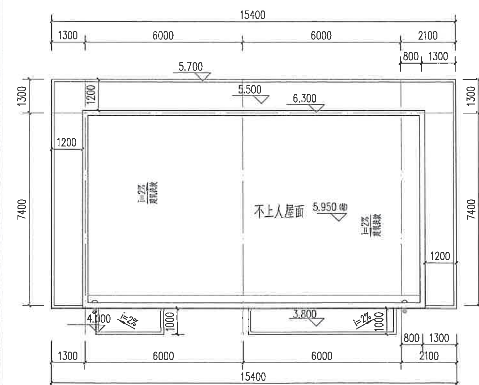
污水处理用房 屋面层平面图 1:100
