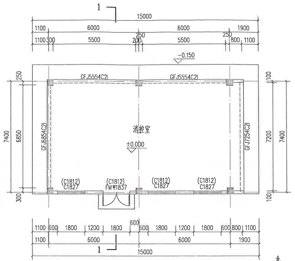
消控室 一层平面图:100 消防控制室面积99平方米
