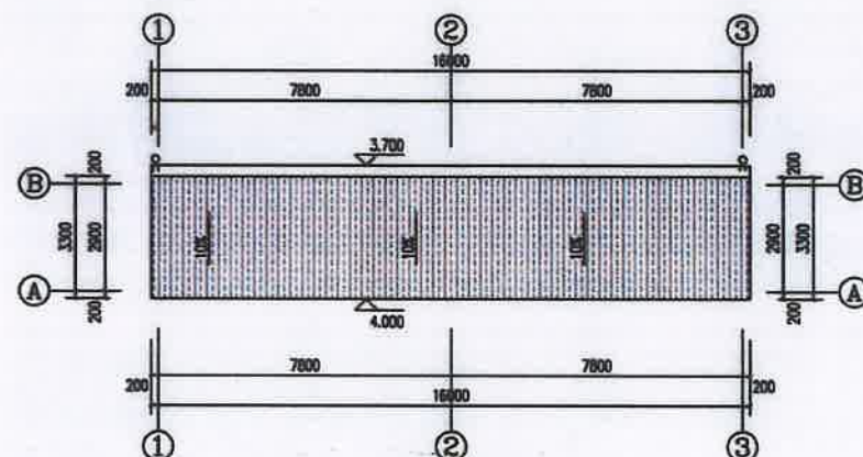
連雨棚屋面平面圖 1:100
