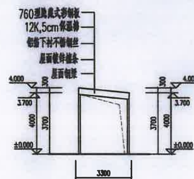
1-1 1:100
