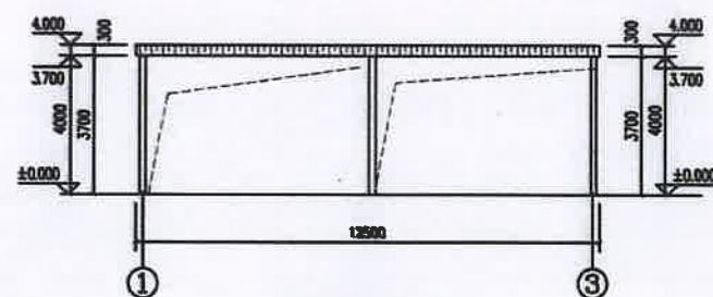
①~③轴立面 1:100
