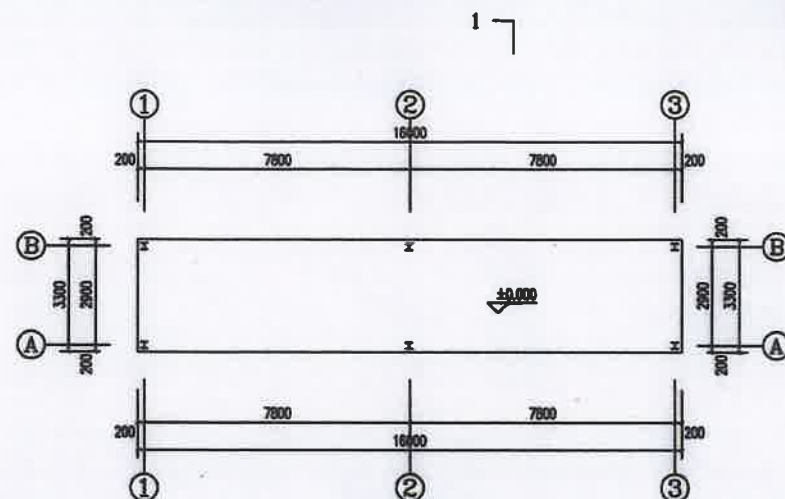
這兩相一層平面圖 1:100
