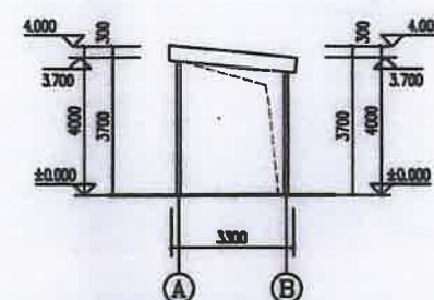
①~③轴立面图 1:100
