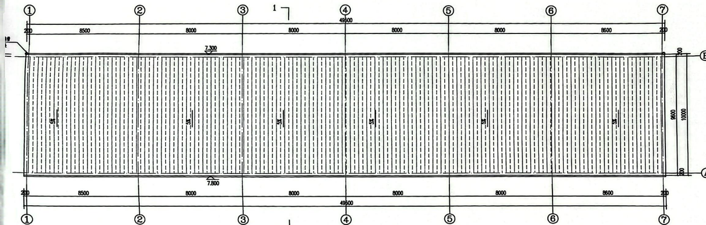
遮雨棚屋面平面图 1:100
