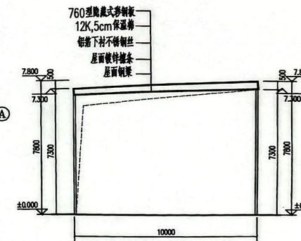
B-A 轴立面图 1:100
