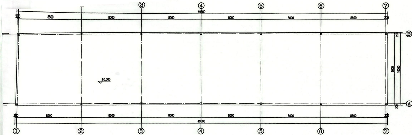
遮雨棚一层平面图 1:100
