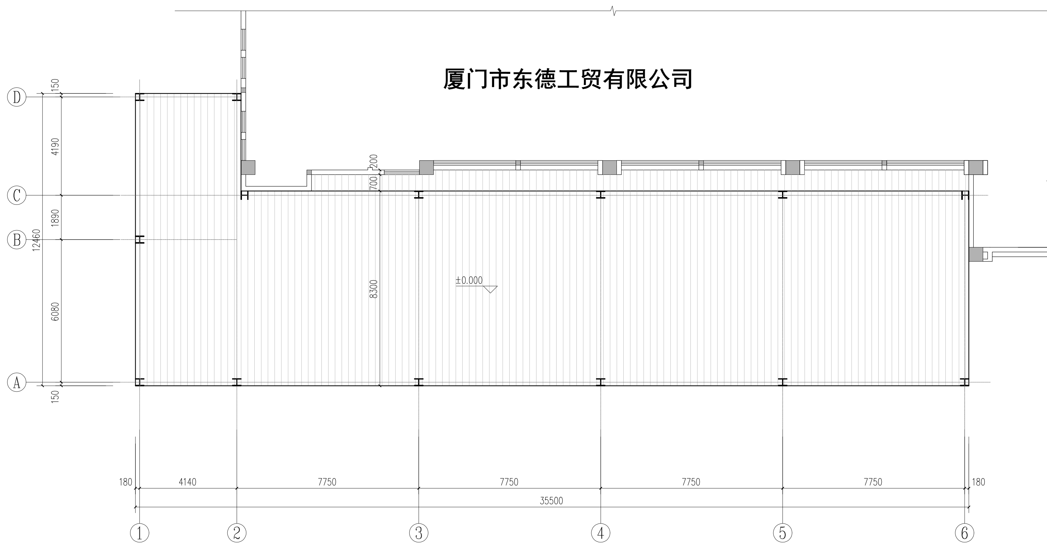
一层平面图
