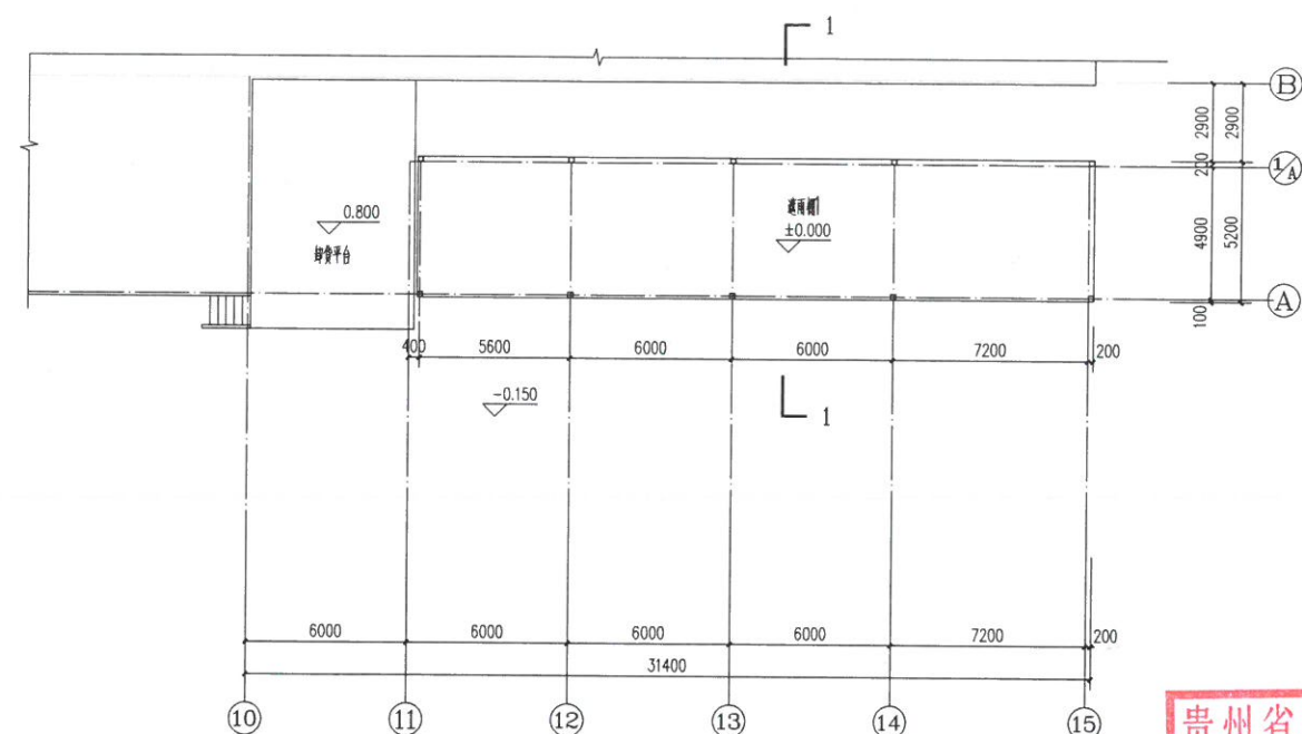
遮雨棚1—层平面图 1:150
