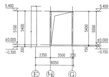
①E-①G轴立面图 1:150
