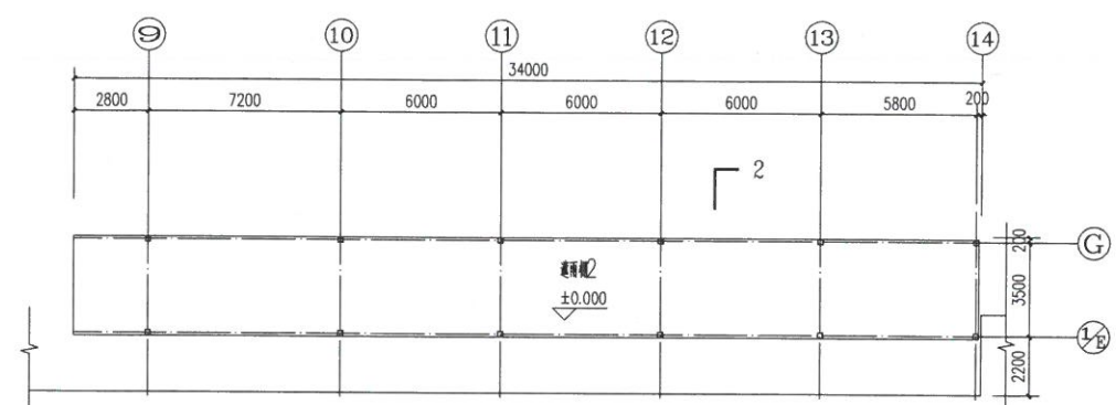
遮雨棚2一层平面图 1:150
