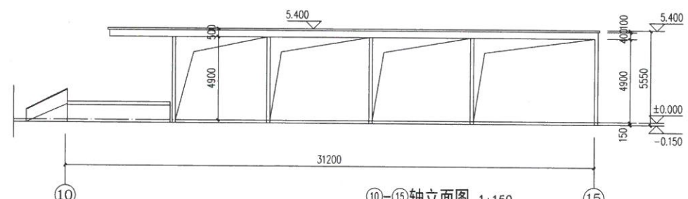
⑩-⑮轴立面图 1:150
