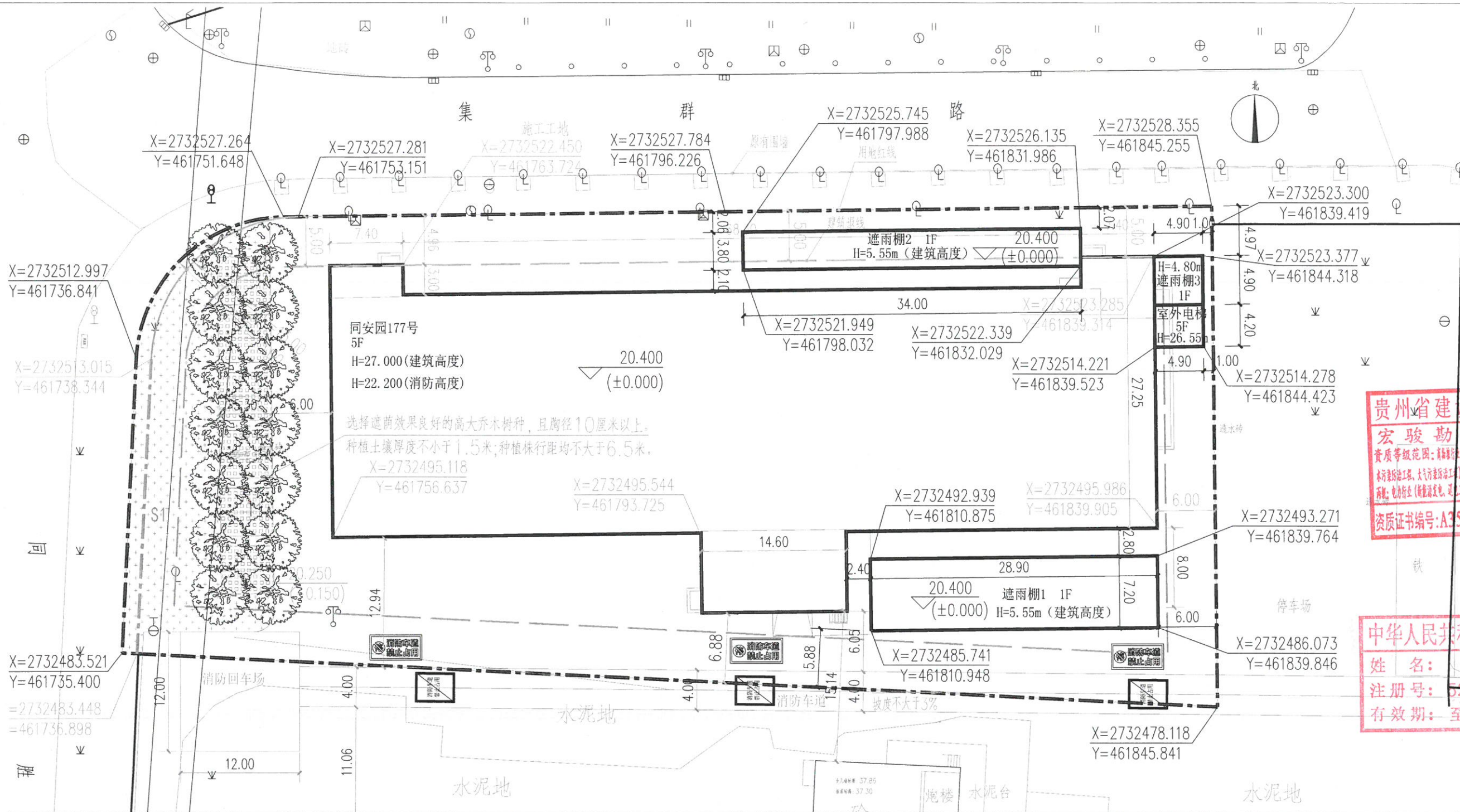
总平面图 1:500
