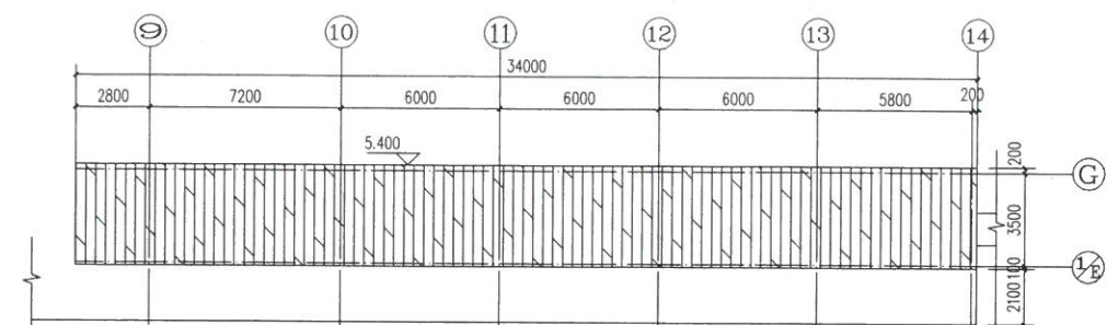
遮雨棚2屋面层平面图 1:150
