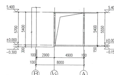
①A-①A轴立面图 1:150
