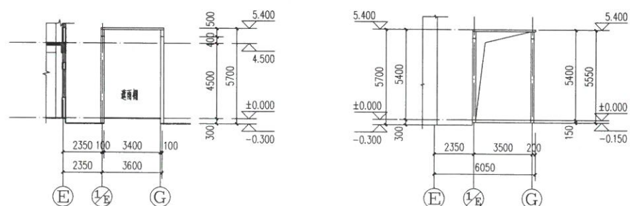
2-2 剖面图 1:150
