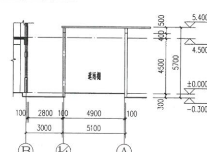
1-1 剖面图 1:150
